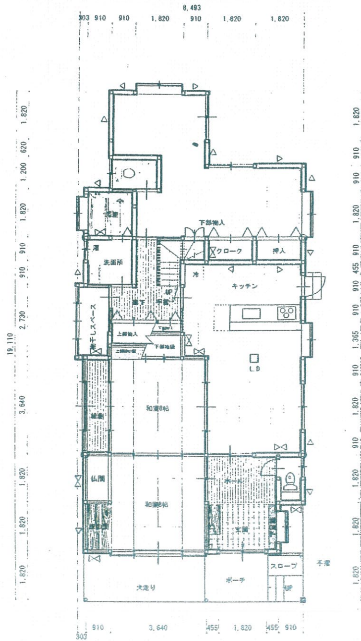
1階平面図 SCALE 1 : 100
